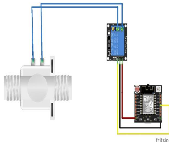
Gambar 4. Rangkaian Perangkat Keras
