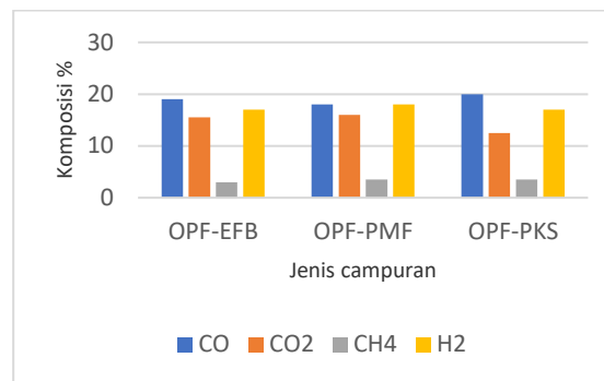
Gambar 6. Komposisi Syn-gas dari Campuran OPF-EFB, OPF-PMF, dan OPF-PKS (Moni dkk., 2018)
